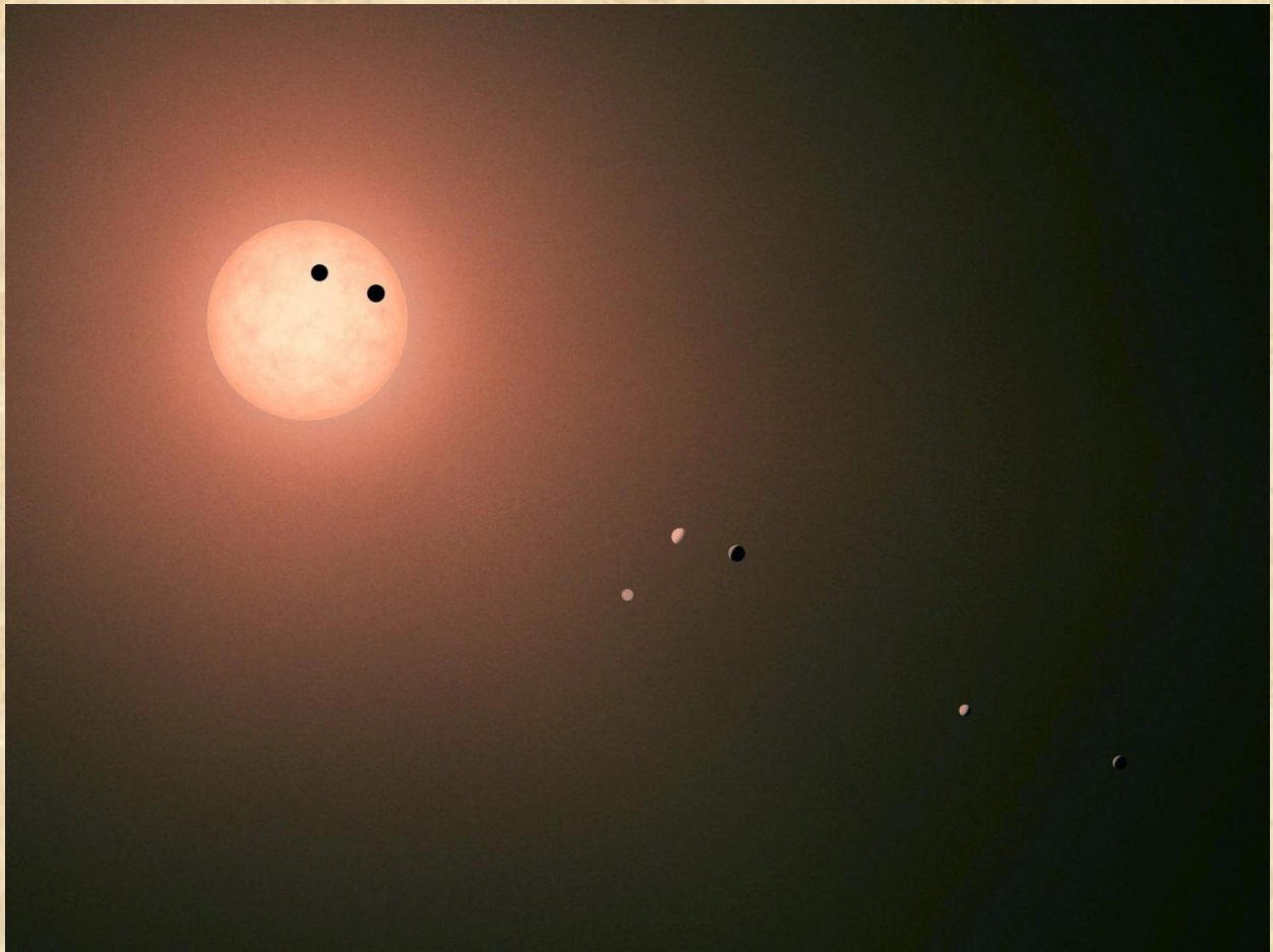
trappist-1
